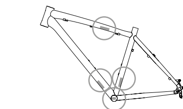
Fig. 9 Amplasare posibilă a plăcuței de identificare
