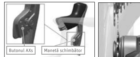
Fig. 93 Aliniere role schimbător ©Shimano
