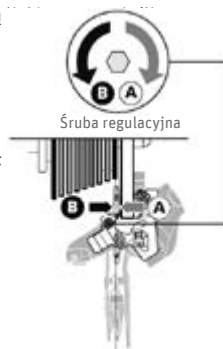
Rys. 82 Obróć górną śrubę regulacyjną ©Shimano
