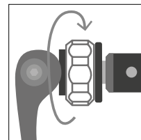
Afb. 123 Voorspanning verhogen
