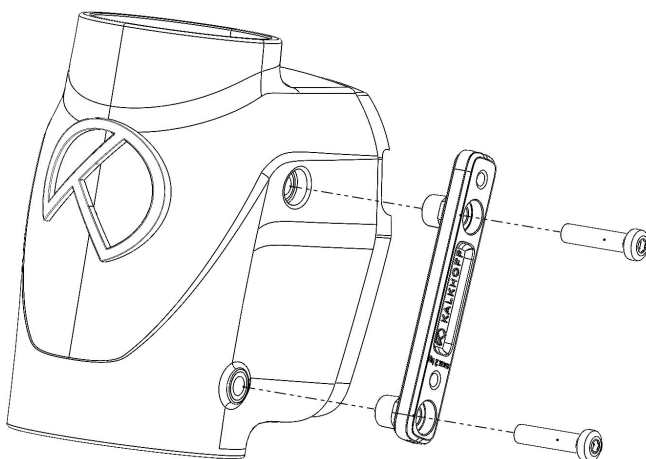
Abb. 35 Adapterplatte montieren
