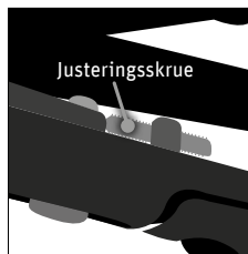
Fig. 110 Drejning af justeringsskruer
