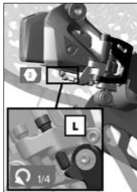
Fig. 91 Anslagsskruer L ©Sram
