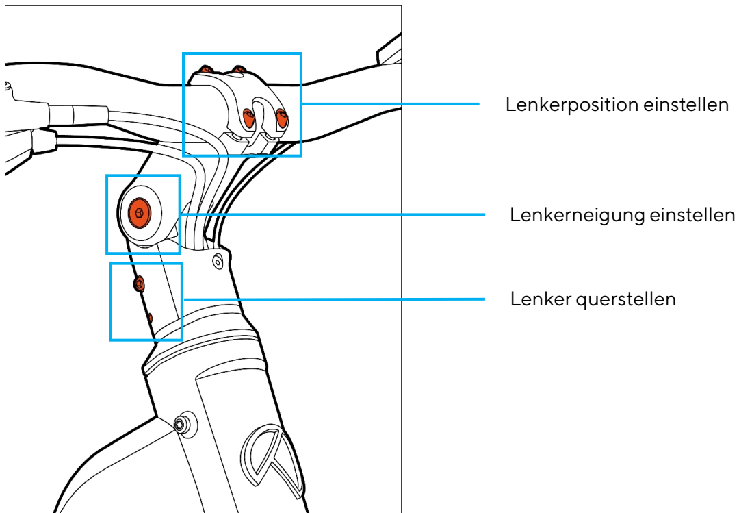
Abb. 58 Einstellschrauben Vorbau Aluminium, verstellbar
