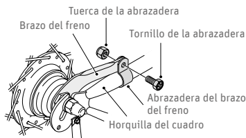
Fig. 136 Fijar el brazo del freno ©Shimano
