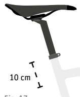
Fig. 17 Mindste indføringsdybde
