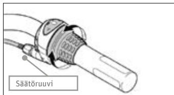
Kuva 100 Shimano-vakiokiertoakahva ©Shimano
