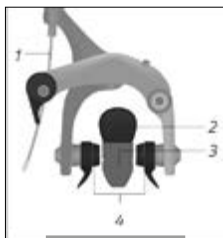
Hamulec linkowy
