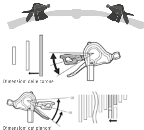
Fig. 69 Passare a una marcia inferiore ©Shimano
