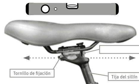
Fig. 25 Ajustar posición del asiento
