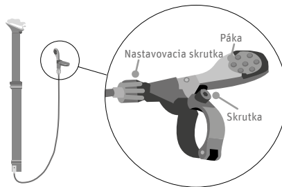
Obr. 20 Spúšťacia sedlovka
