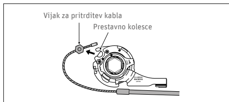
Sl. 132 Odstranitev vijaka za pritrditev kabla ©Shimano
