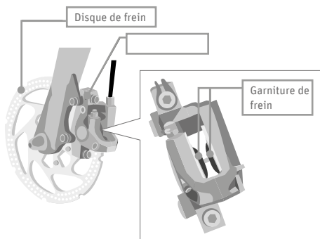
Fig. 45 Frein à disque ©Shimano
