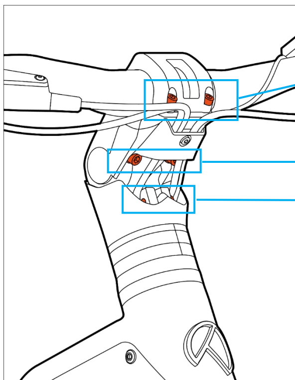
Abb. 56 Einstellschrauben Cockpit 2.0
