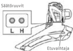
Kuva 84 Säätöruuvi ©Shimano
