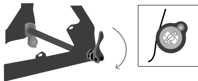
Obr. 121 Otočení páky ve směru hodinových ručiček
