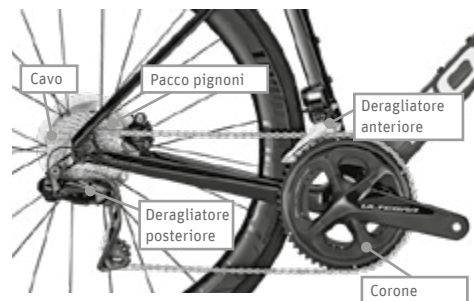
Fig. 63 Deragliatore elettronico
