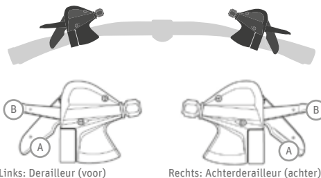
Afb. 64 Shimano standaard-versnellingshendel ©Shimano
