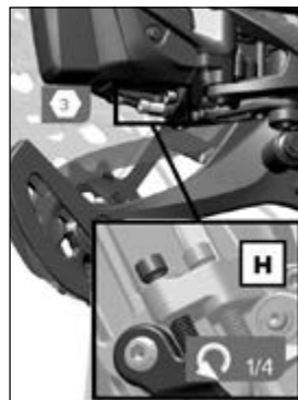
Fig. 92 Anslagsskruer H ©Sram
