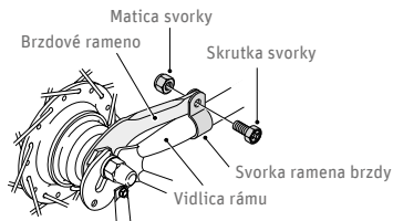
Obr. 136 Upevnenie ramena brzdy ©Shimano
