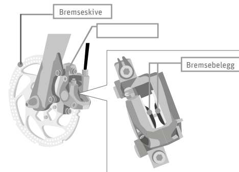
Fig. 45 Skivebrems ©Shimano
