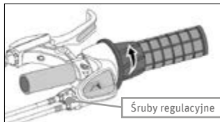
Rys. 101 Przelatczanie na niższy bieg ©Shimano
