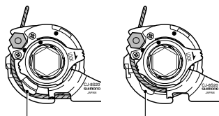
Obr. 141 Kontrola vedenia kábla ©Shimano
