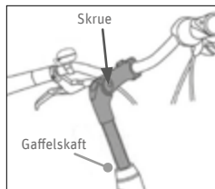
Fig. 31 Skafststyre festem vinkeljusterbar
