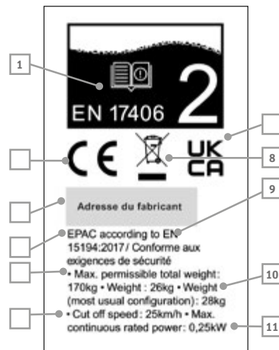
Fig. 8 Plaque signalétique
