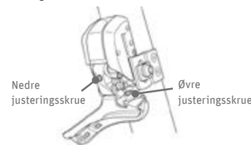
Fig. 89 Justeringssskruer ©Shimano
