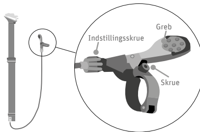
Fig. 20 Sænkbar sadelpind
