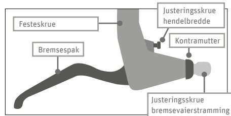
Fig. 46 Bremsehåndtak
