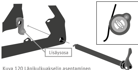
Kuva 120 Läpikulkuakselin asentaminen
