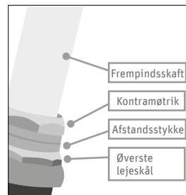
Fig. 35 Gevindstyrsæt
