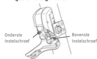
Afb. 89 Instelschroeven ©Shimano
