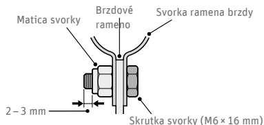
Obr. 137 Montáž svorky ramena brzdy ©Shimano
