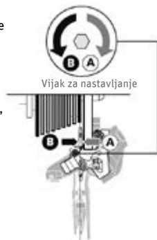
Sl. 82 Obračanje zgornjega vijaka za nastavljanje ©Shimano
