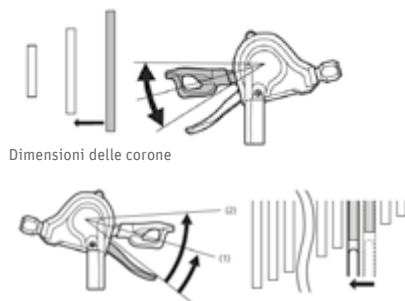
Dimensioni dei pignoni
