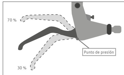
Fig. 50 Recomendación de ajuste del punto de presión
