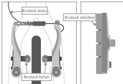
Obr. 51 Ráfková brzda
