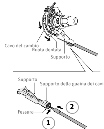
Fig. 140 Inserimento del cavo nella fessura ©Shimano
