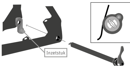
Afb. 120 Steekas aanbrengen
