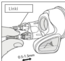
Rys. 106 Lekko pociągnij za linki ©Shimano
