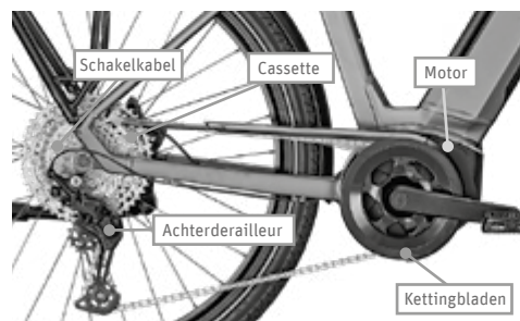
Afb. 62 Mechanische kettingschakeling
