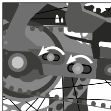
Sl. 109 Odvijanje vijakov
