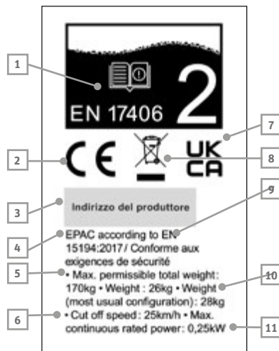
Fig. 8 Targhetta identificativa
