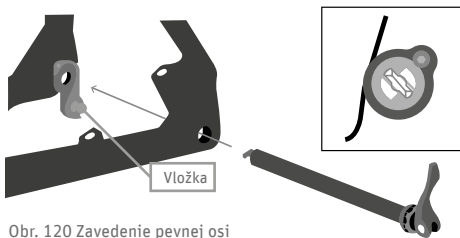
Obr. 120 Zavedenie pevnej osi
