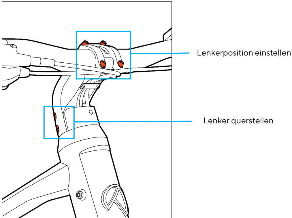
Abb. 59 Einstellschrauben Vorbau Aluminium, integriert, starr
