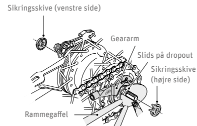
Fig. 134 Monter sikringsskiver ©Shimano
