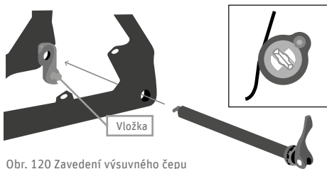
Obr. 120 Zavedení výsuvného čepu
