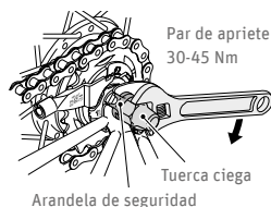
Fig. 135 Fijar la rueda ©Shimano
