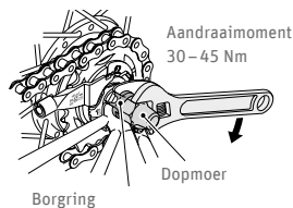
Afb. 135 Wiel bevestigen ©Shimano
