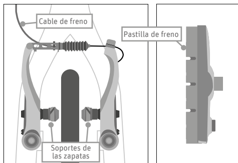
Fig. 51 Freno de llanta
