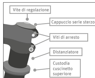
Fig. 36 Attacco Ahead I
