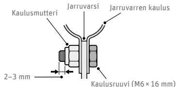
Kuva 137 Jarruvarren kauluksen asennus ©Shimano
