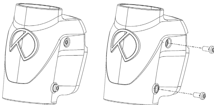
Abb. 34 Schrauben entnehmen
