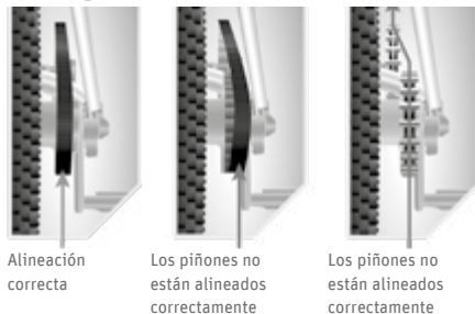
Fig. 108 Alineación de la correa ©Gates
