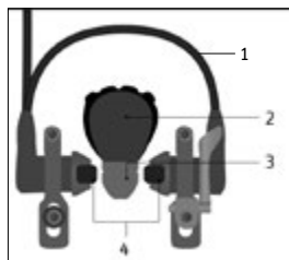
Fig. 43 Frenos hidráulicos de llanta (ejemplo)
