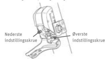
Fig. 89 Indstillingsskruer ©Shimano
