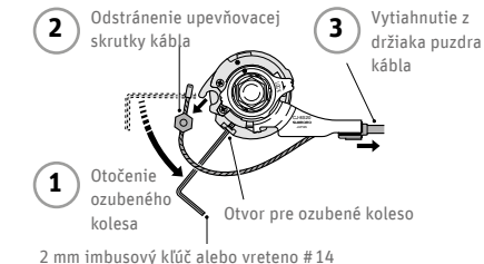
Obr. 131 Típ: odstránenie puzdra kábla ©Shimano
