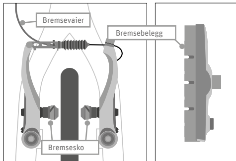
Fig. 51 Felgbrems
