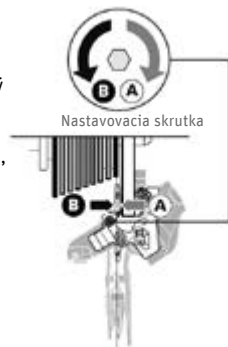
Obr. 82 Otočenie hornej nastavovacej skrutky ©Shimano
