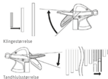
Fig. 65 Skift til et højere gear ©Shimano
