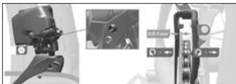
Fig. 96 Justering av øvre anslag ©Sram
