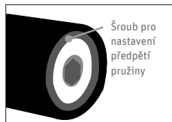
Obr. 22 Odpřužená sedlovka
