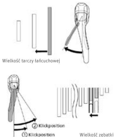
Rys. 72 Przelączenie na niższy bieg ©Shimano
