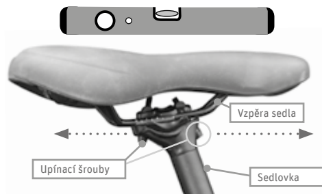
Obr. 24a Nastavení posedu
