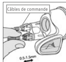
Fig. 106 Tirer légèrement sur les câbles de commande ©Shimano
