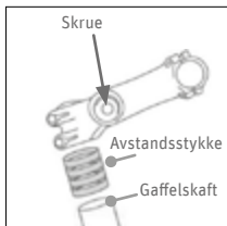
Fig. 32 Ahead-styrestem vinkeljusterbar
