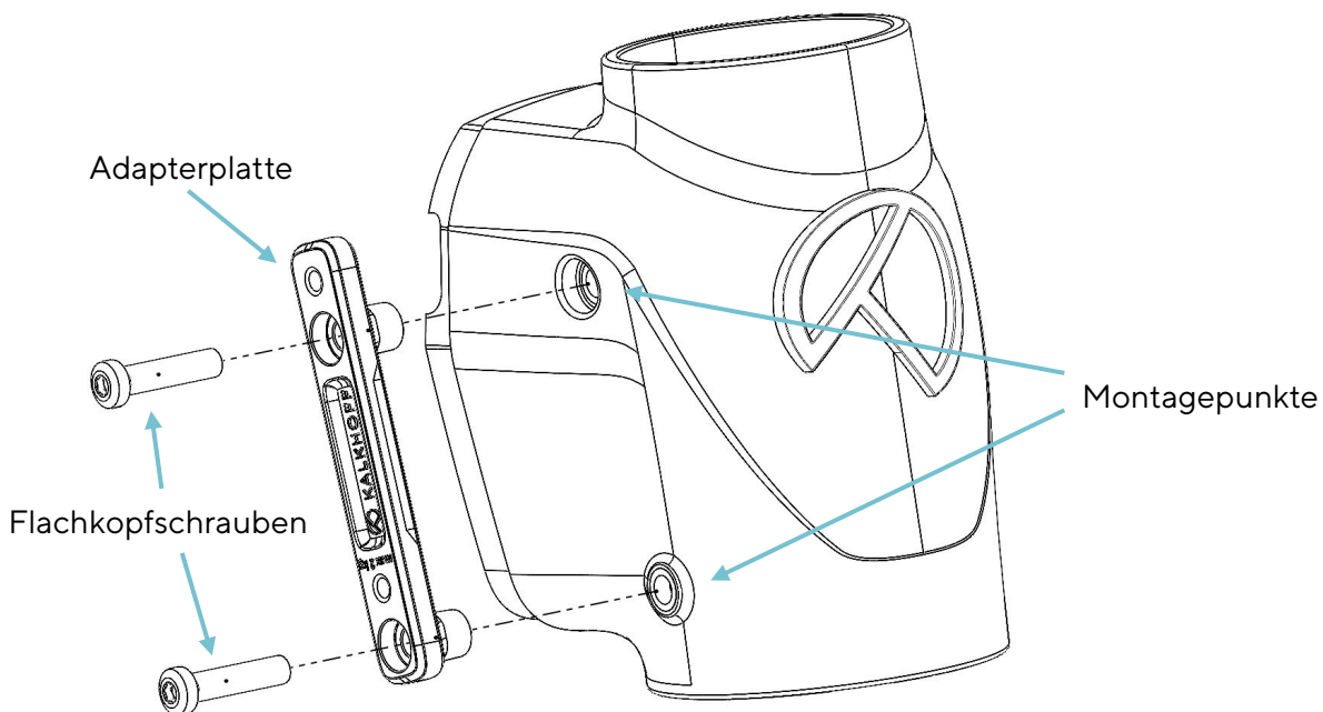
Abb. 32 Flachkopfschrauben, Adapterplatte, Montagepunkte
