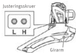
Fig. 84 Justeringssskruer ©Shimano
