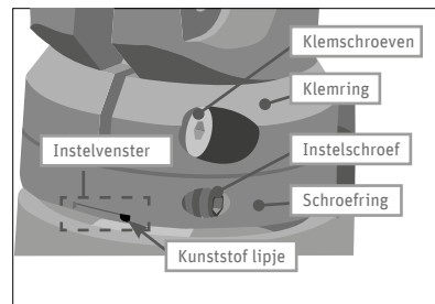
Afb. 37 Ahead-balhoofd II
