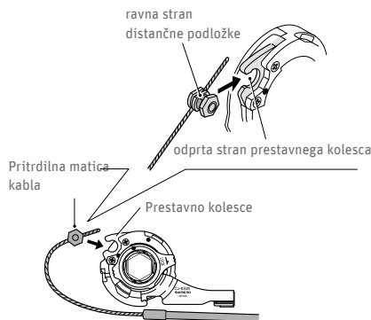
Sl. 138 Namestitev kabla ©Shimano
