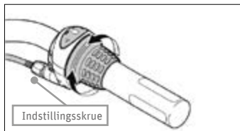
Fig. 100 Shimano-standarddrejeregreb ©Shimano
