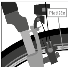
Sl. 39 Zavora na platišču
