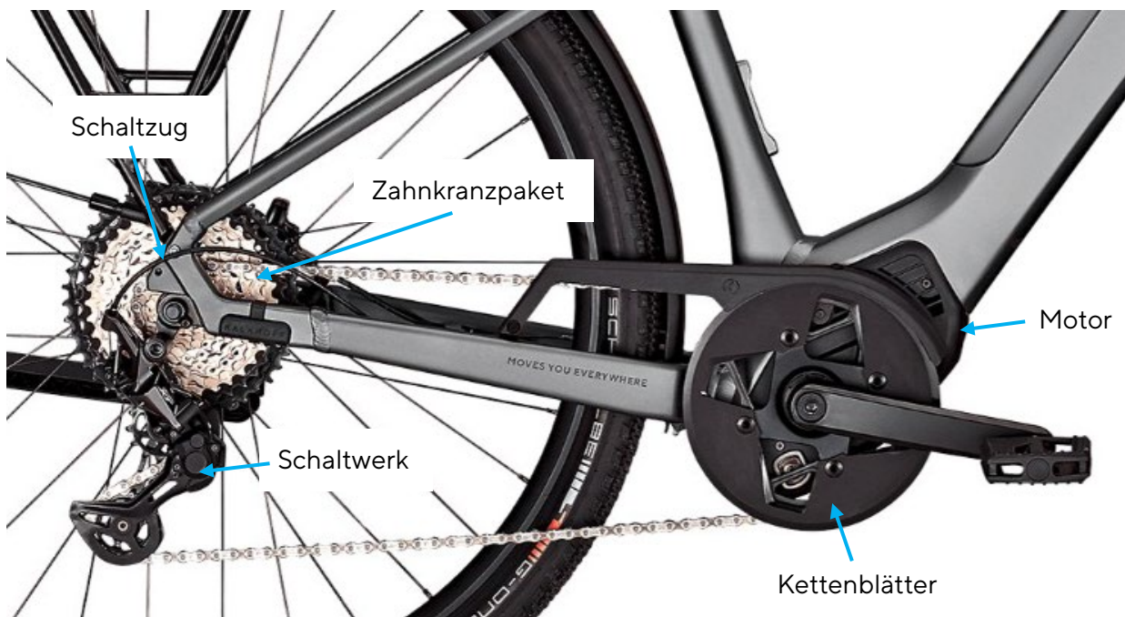
Abb. 86 Mechanische Kettenschaltung
