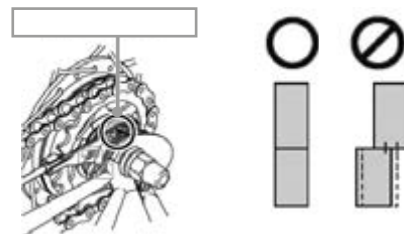
Kuva 103 Merkkiviivojen kohdistuksen tarkistus ©Shimano
