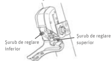
Fig. 89 Șuruburi de reglare ©Shimano
