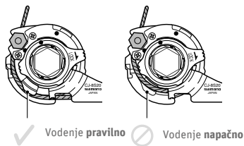
Sl. 141 Kontrola napeljave kablov ©Shimano
