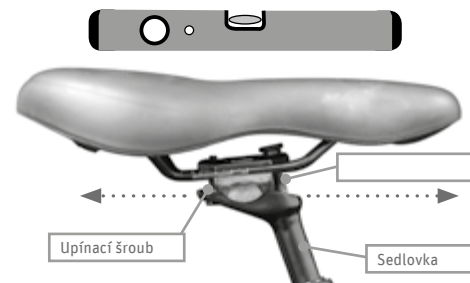
Obr. 25 Nastavení posedu
