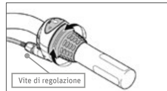
Fig. 100 Manopola Shimano Standard ©Shimano
