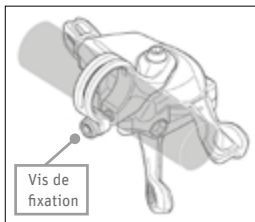
Fig. 59 Module de commande de Shimano ©Shimano
