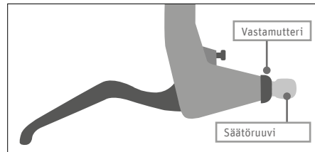
Kuva 55 Jarruvaijerin kiristysten säätöruuvi
