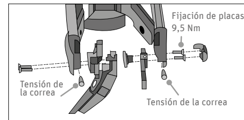
Fig. 113 Ajustar la tensión de la correa
