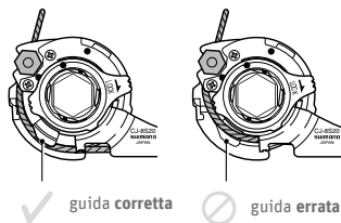
Fig. 141 Controllo della posa cavi ©Shimano
