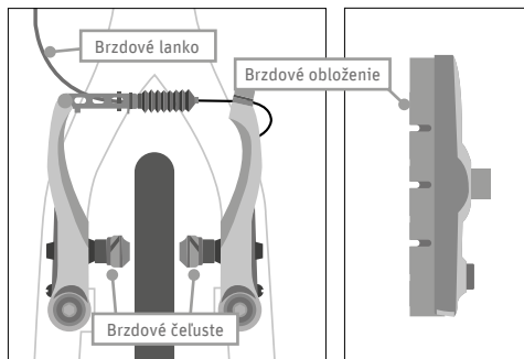
Obr. 51 Ráfiková brзда
