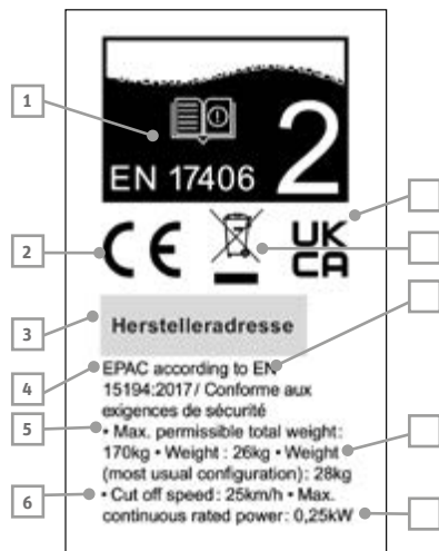
Rys. 8 Tabliczka znamionowa
