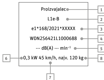
Sl. 10 Tovarniška ploščica
