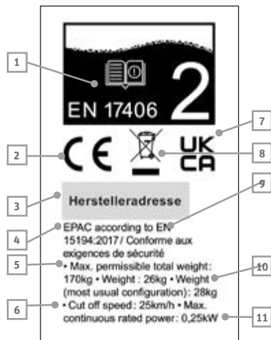
Obr. 8 Typový štítek
