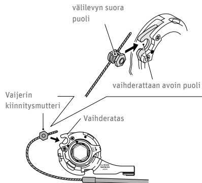
Kuva 138 Vaijerin kiinnitys ©Shimano
