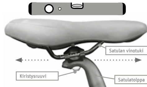
Kuva 23 Istuma-asennon säätäminen
