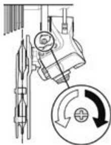
Fig. 85 Justeringssskruer ©Shimano
