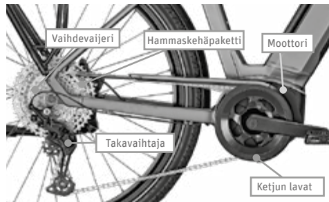
Kuva 62 Mekaaninen ketjuvaihteisto
