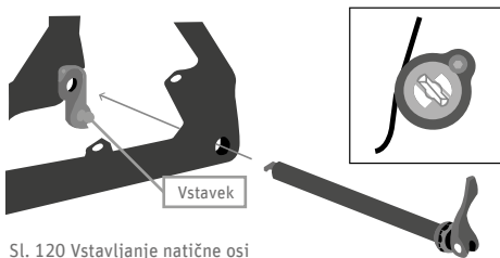
Sl. 120 Vstavljanje natične osi
