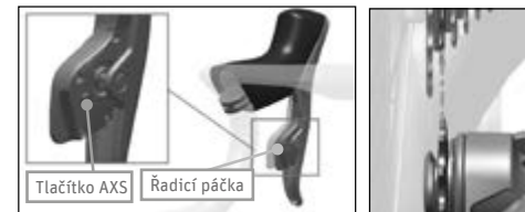
Obr. 93 Vyrovnání řadičí kladičky ©Sram
