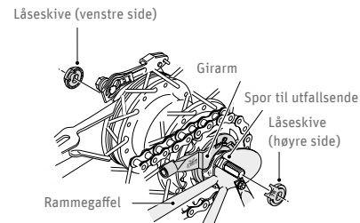
Fig. 134 Montere låseskiver ©Shimano
