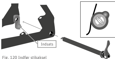
Fig. 120 Indfør stikaksel
