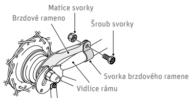
Obr. 136 Upevnění brzdového ramena ©Shimano
