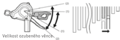
Obr. 68 Přepnutí na vyšší převod ©Shimano
