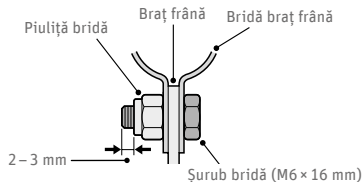
Fig. 137 Montaj bridă brat frână ©Shimano
