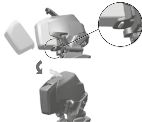
Kuva 81 Akun asentaminen ©Sram
