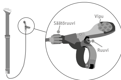
Kuva 20 laskettava satulatulppa
