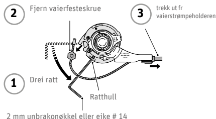
Fig. 131 Tips fjerne vaierhylse ©Shimano
