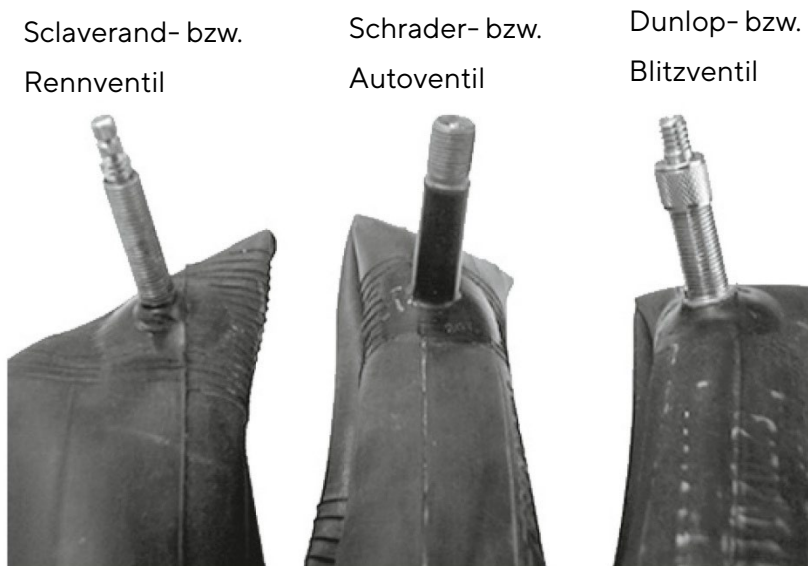
Abb. 112 Verschiedene Ventiltypen
