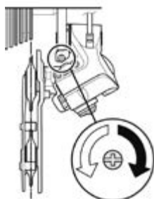
Obr. 85 Nastavovacia skrutka ©Shimano
