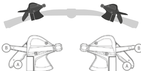
Obr. 64 Standardní řadicí páčka Shimano ©Shimano
