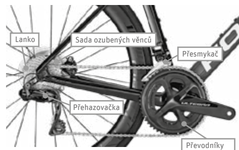
Obr. 63 Elektronické řetězové řazení
