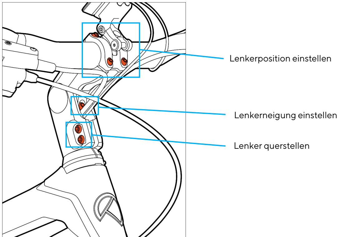
Abb. 57 Einstellschrauben Concept EX, verstellbar
