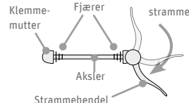
Fig. 116 Hurtigutløser på hjul
