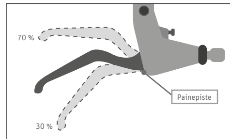
Kuva 50 Suositeltu painepisteasetus
