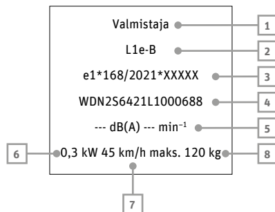
Kuva 10 Tehdaskilpi
