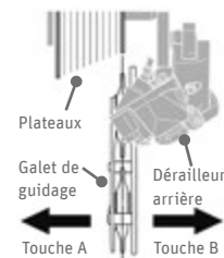
Fig. 88 Réglage du dérailleur arrière ©Shimano
