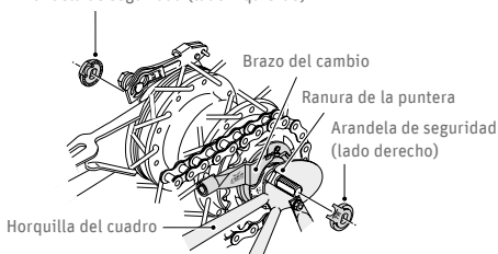
Fig. 134 Montar las arandelas de seguridad ©Shimano
