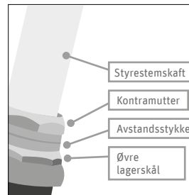
Fig. 35 Gjenget styresett
