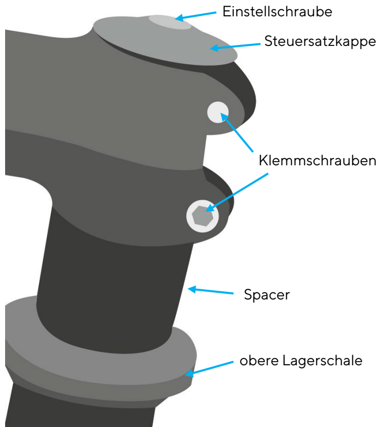
Abb. 73 Ahead-Steuersatz I
