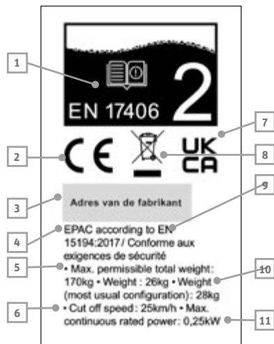
Afb. 8 Typeplaatje
