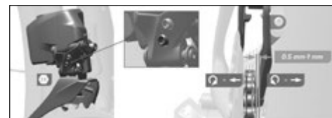
Fig. 97 Réglage de la butée supérieure ©Sram
