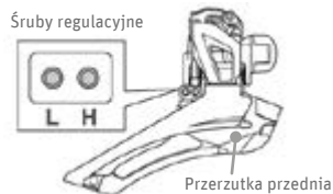
Rys. 84 Śruby regulacyjne ©Shimano
