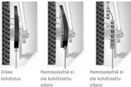
Kuva 108 Hihnan säätö ©Gates
