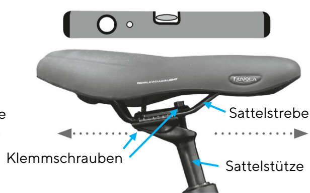
Abb. 51 Sitzposition einstellen
