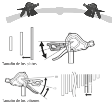
Fig. 69 Cambiar a una marcha más baja ©Shimano
