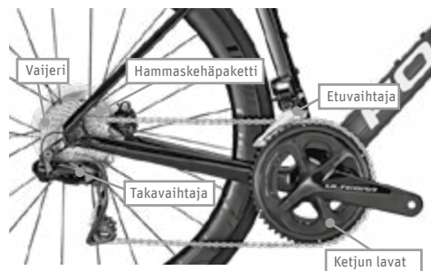
Kuva 63 Elektroninen ketjuvaihteisto
