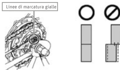
Fig. 103 Controllare allineamento delle linee di marcatura ©Shimano
