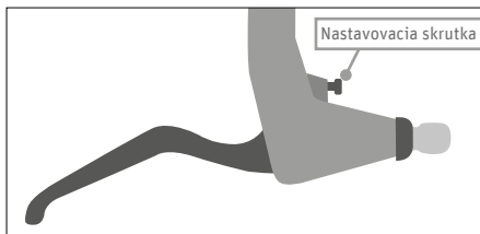
Obr. 49 Nastavovacia skrutka dráhy páčky
