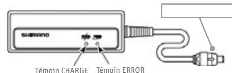
Fig. 74 Chargeur ©Shimano
