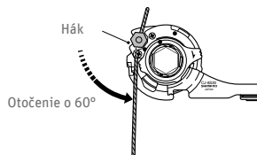
Obr. 139 Otočenie kábla doprava ©Shimano
