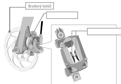
Obr. 45 Kotúčová brzda ©Shimano
