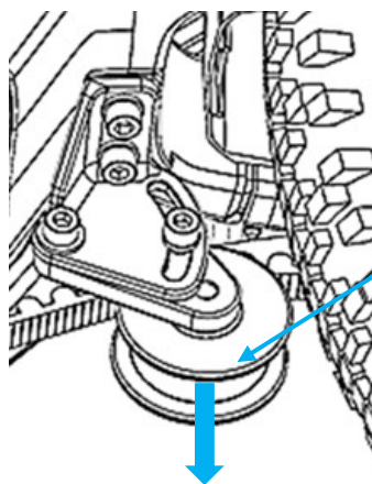
Abb. 101 Riemen Spannung erhöhen
