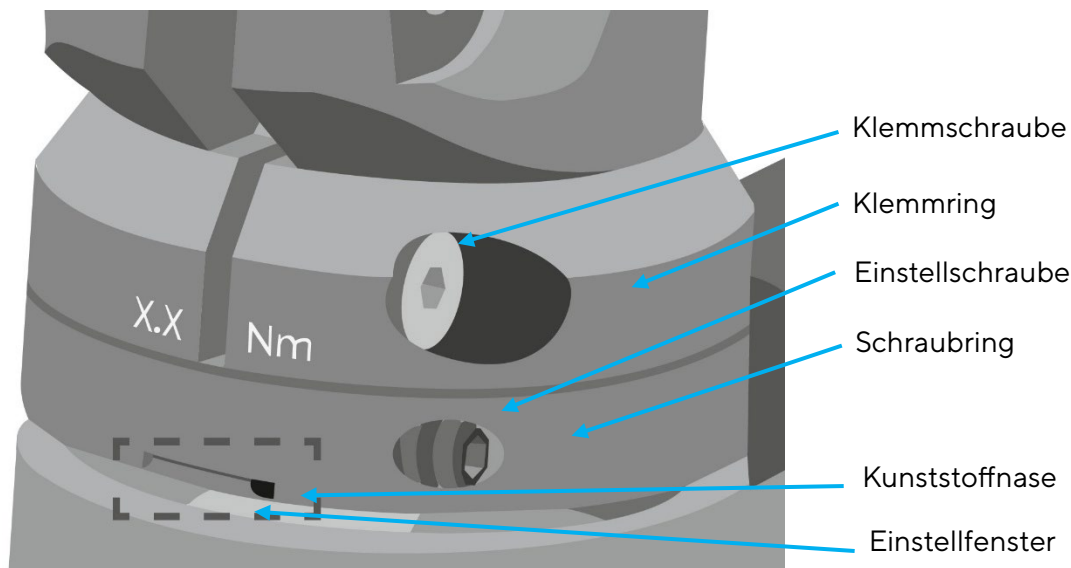
Abb. 74 Ahead-Steuersatz II
