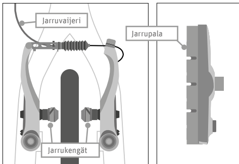
Kuva 51 Vanejarru
