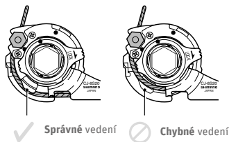
Obr. 141 Kontrola uložení lanka ©Shimano
