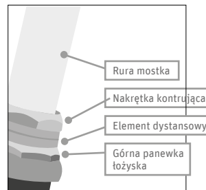
Rys. 35 Stery gwintowane
