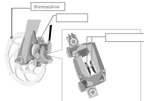
Fig. 45 Skivebremse ©Shimano
