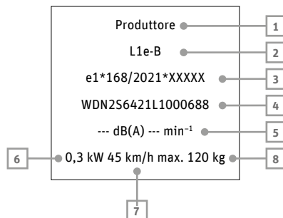
Fig. 10 Targhetta del produttore
