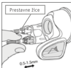
Sl. 106 Rahlo vlečenje prestavnih žic ©Shimano
