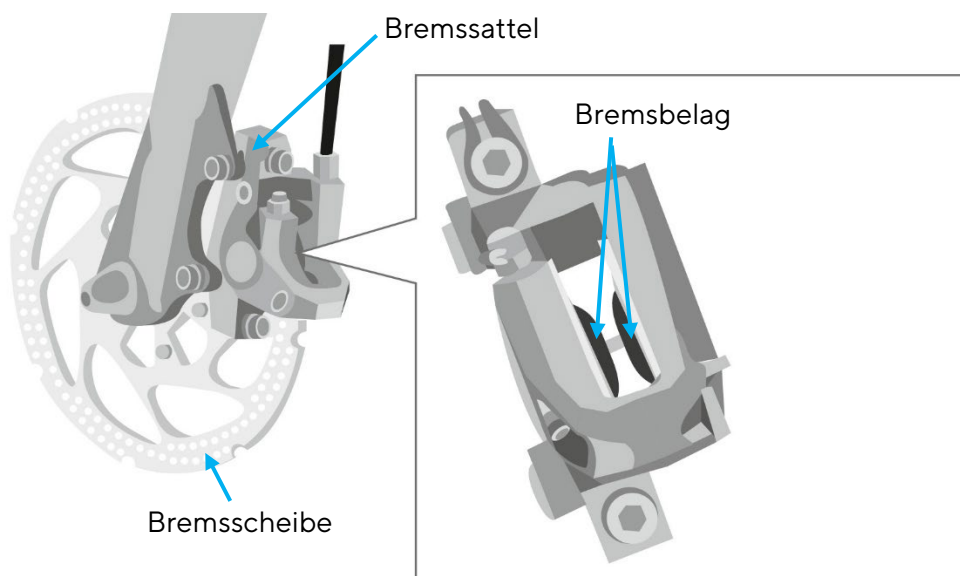
Abb. 78 Scheibenbremse @Shimano
