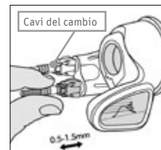
Fig. 106 Leggera trazione dei cavi del cambio ©Shimano
