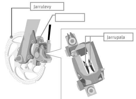
Kuva 45 Jarrulevy ©Shimano
