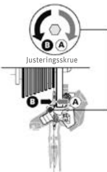
Fig. 82 Vri den øvre justeringsskruen ©Shimano
