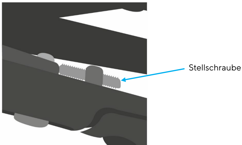
Abb. 96 Stellschraube drehen
