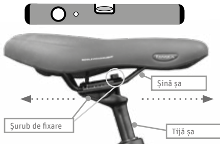
Fig. 24b Reglarea poziției de ședere
