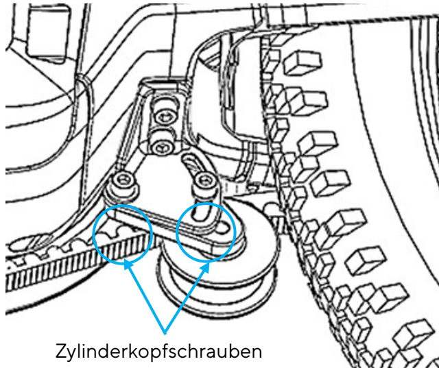
Abb. 100 Zylinderkopfschrauben lösen
