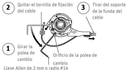
Fig. 131 Consejo: quitar la funda del cable ©Shimano
