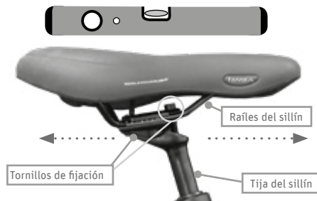
Fig. 24b Ajustar posición del asiento
