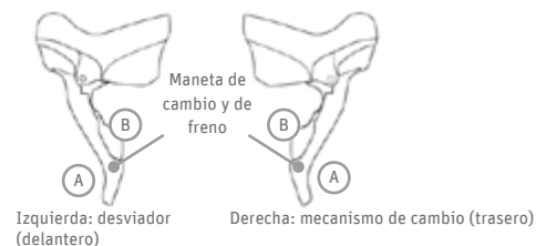
Fig. 70 Dual Control de Shimano ©Shimano
