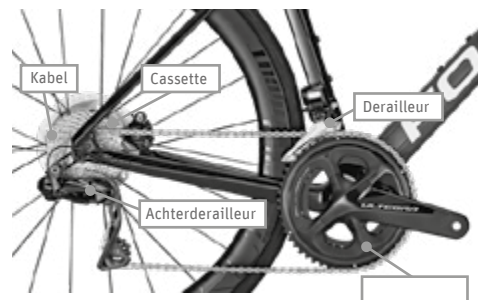
Afb. 63 Elektronische kettingschakeling
