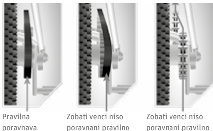
Sl. 108 Izravnava jermena ©Gates
