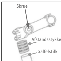
Fig. 32 Ahead-frepind vinkeljusterbar
