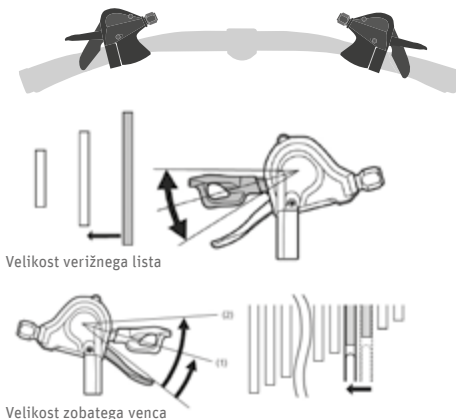
Sl. 69 Prestavljanje za nižjo prestavo ©Shimano
