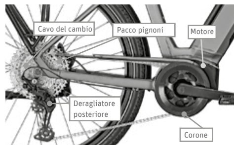
Fig. 62 Deragliatore meccanico
