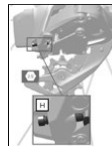
Fig. 95 Vite di arresto H ©Sram
