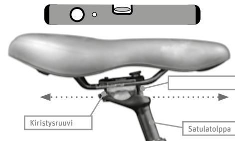
Kuva 25 Istuma-asennon säätäminen
