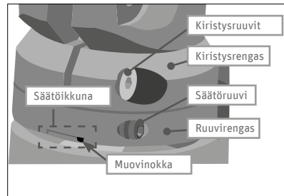
Kuva 37 Ahead-ohjainsarja 2
