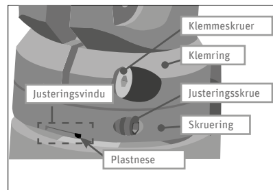
Fig. 37 Ahead-styresett II
