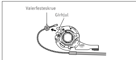
Fig. 132 Fjern vaierfesteskruen ©Shimano
