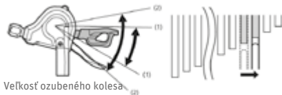
Obr. 68 Preradenie na vyšší stupeň ©Shimano
