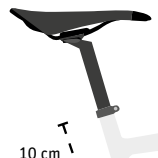
Afb. 17 Minimum insteekdiepte
