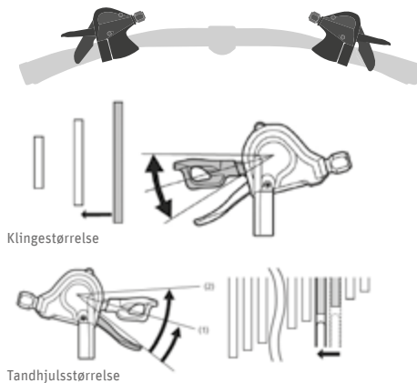
Fig. 69 Skift til et lavere gear ©Shimano
