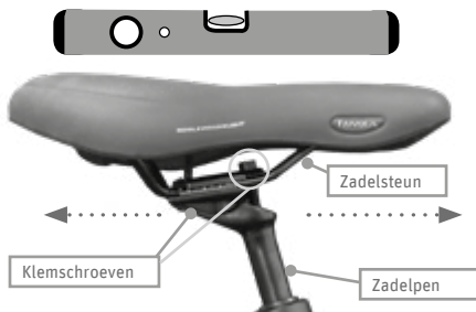
Afb. 24b Zitpositie instellen
