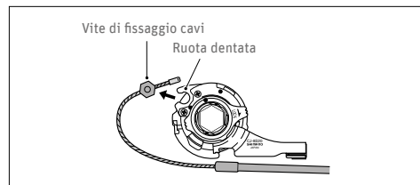
Fig. 132 Rimozione vite di fissaggio cavi ©Shimano
