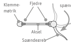
Fig. 116 Hurtigspænder på hjul
