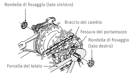
Fig. 134 Montaggio rondelle di fissaggio ©Shimano
