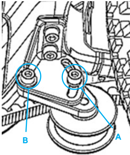
Abb. 103 Zylinderkopfschrauben anziehen
