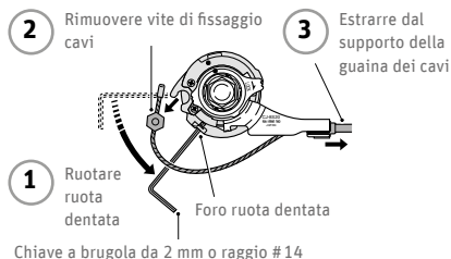
Fig. 131 Consiglio per rimozione guaina dei cavi ©Shimano
