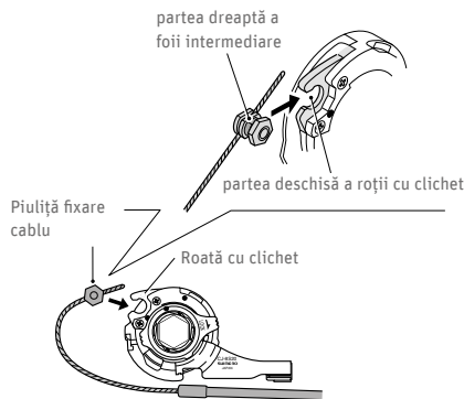
Fig. 138 Montati cablul ©Shimano
