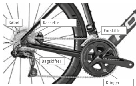
Fig. 63 Elektronisk kædeskifte
