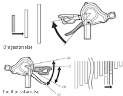
Fig. 68 Skift til et højere gear ©Shimano
