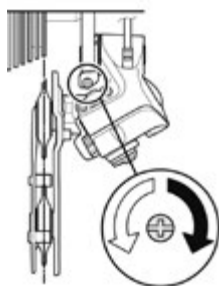
Fig. 85 Tornillo de ajuste ©Shimano
