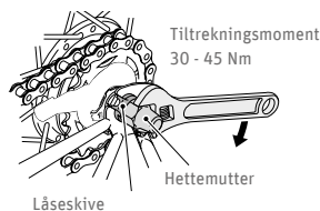
Fig. 135 Feste hjul ©Shimano
