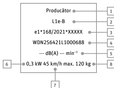
Fig. 10 Plăcuța producătorului
