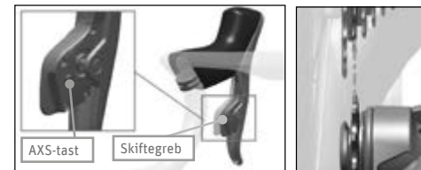
Fig. 93 Placering af skifteruller ©Sram
