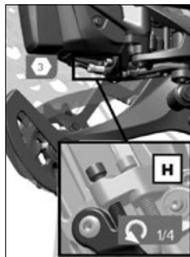
Afb. 92 Aanslagschroef H ©Sram
