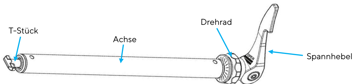
Abb. 109 R.A.T.-Steckachse
