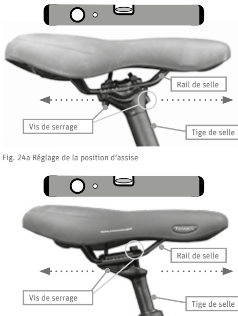
Fig. 24b Réglage de la position d'assise
