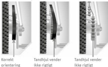
Fig. 108 Justering af rem ©Gates
