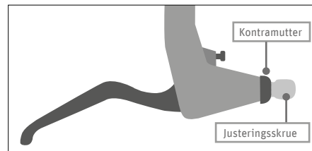
Fig. 55 Justeringsskru bremsevaierstramming
