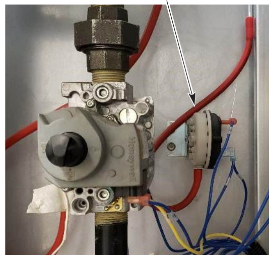
Pressostat de la hotte d'évacuation
