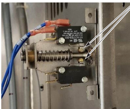
Rouleaux du contacteur de porte
