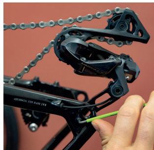
2. Colocar la Tuerca FOCUS de eje pasante (3).
