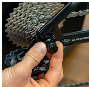
6. Atornilla el casquillo roscado (2d) en la tuerca FOCUS de eje pasante por el lado de la transmisión.
