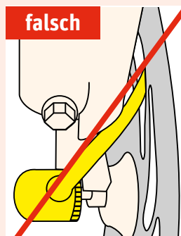
Schnellspannhebel und Bremscheibe kollidieren
