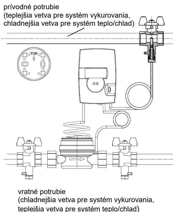
Obr.. 1: PolluCom F v systéme vykurovania PolluCom FH v systéme teplo/chlad
