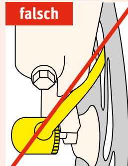
Schnellspannhebel und Bremsscheibe kollidieren
